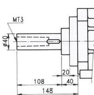
FD65-100-MT3
