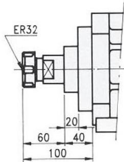
FD65-100-MT3
