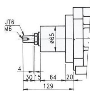
FD65-100-JT6
